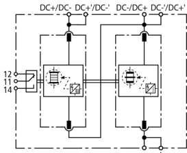
Schemat połączeń DSE M 2P 60 FM
