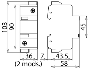
Rysunek wymiarowy DG 1000
