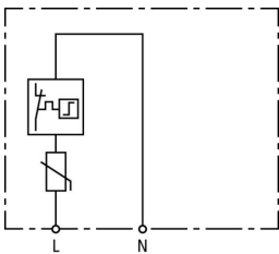
Schemat połączeń DCOR L 1P 275
