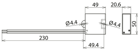
Rysunek wymiarowy DCOR L 1P 275
