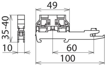
Rysunek wymiarowy SH1 18X3 ST
