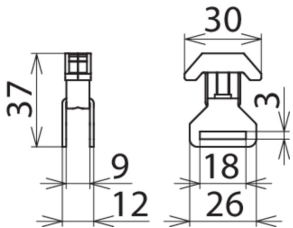
Rysunek wymiarowy AK 35 SN 18X3 GG
