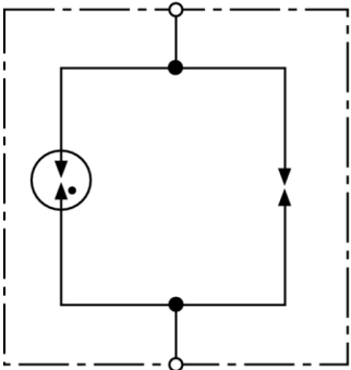
Schemat połączeń SDS 2
