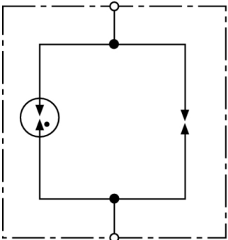
Schemat połączeń SDS 4
