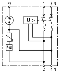
Schemat połączeń SPD+POP 2 255 C25
