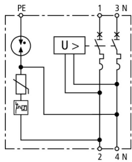
Schemat połączeń SPD+POP 2 255 C32
