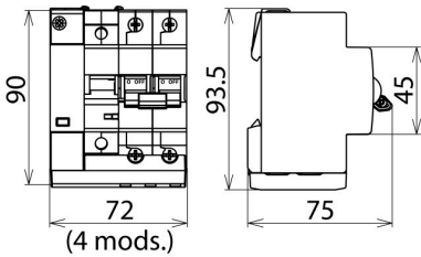
Rysunek wymiarowy SPD+POP 2 255 C32
