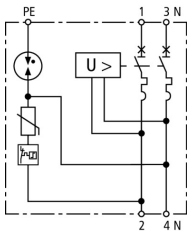
Schemat połączeń SPD+POP 2 255 C40
