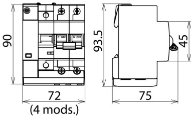
Rysunek wymiarowy SPD+POP 2 255 C40
