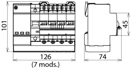
Rysunek wymiarowy SPD+POP 4 255 C63
