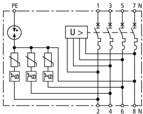
Schemat połączeń SPD+POP 4 255 C63
