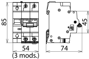
Rysunek wymiarowy POP 2 255 C25
