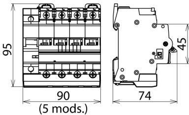
Rysunek wymiarowy POP 4 255 C40
