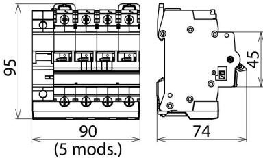
Rysunek wymiarowy POP 4 255 C63
