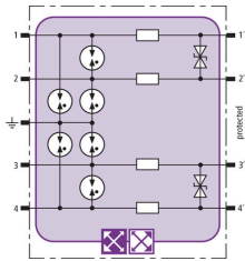
Schemat połączeń BXT ML4 BD EX
