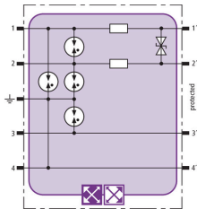
Schemat połączeń BXT ML2 BD S EX 24
