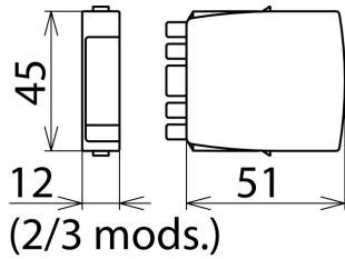
Rysunek wymiarowy BXT ML4 BC EX 24
