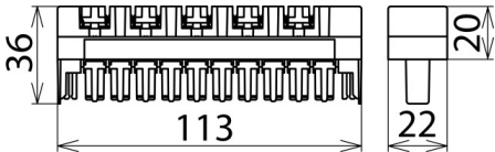
Rysunek wymiarowy BM 10 DRL
