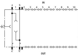
Schemat połączeń BM 10 DRL
