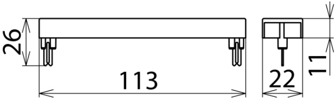
Rysunek wymiarowy EF 10 DRL
