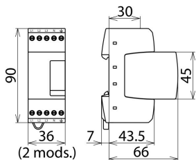
Rysunek wymiarowy DR M 4P 255
