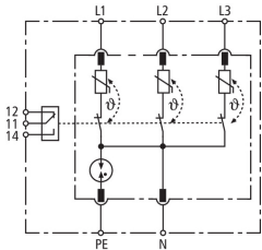
Schemat połączeń DR M 4P 255 SN1872 FM
