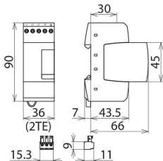
Rysunek wymiarowy DR M 4P 255 SN1872 FM
