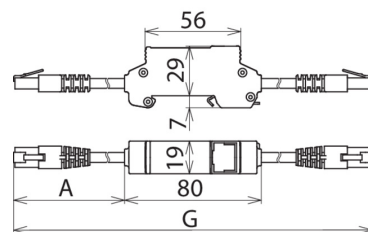
Rysunek wymiarowy DPA M CAT6 RJ45S 48
