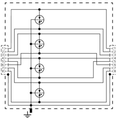
Schemat połączeń DPA M CLD RJ45B 48
