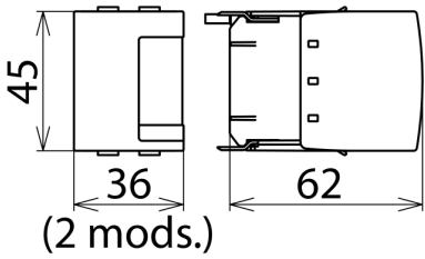
Rysunek wymiarowy DSE MOD 60
