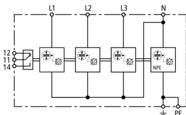
Schemat połączeń DCU EMOB 1 32
