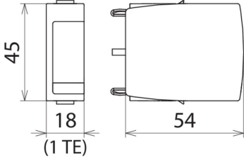
Rysunek wymiarowy DG MOD A NPE
