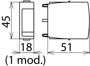
Rysunek wymiarowy DG MOD 600
