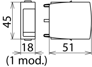
Rysunek wymiarowy DG MOD 75 VA
