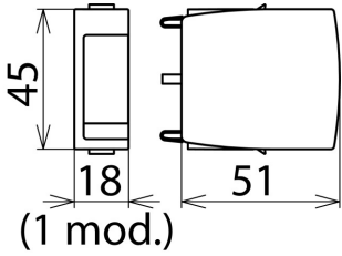
Rysunek wymiarowy DG MOD 275 VA
