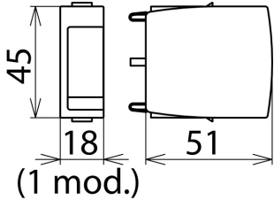
Rysunek wymiarowy DG MOD PV 75
