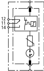
Schemat połączeń DG MOD E H 1000 VA
