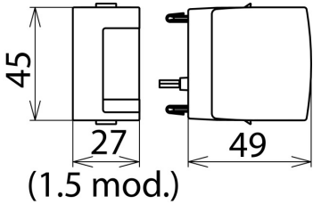
Rysunek wymiarowy DG MOD E DC 60
