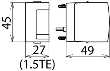
Rysunek wymiarowy DG MOD E DC 242
