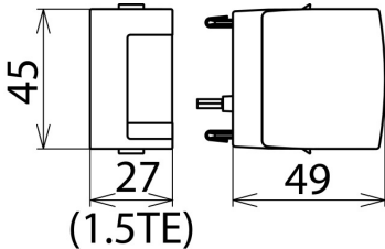
Rysunek wymiarowy DG MOD E DC 550
