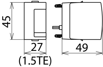
Rysunek wymiarowy DG MOD E DC 900
