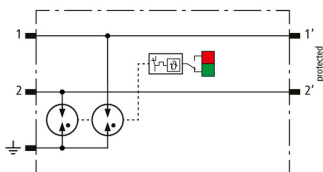
Schemat połączeń BCO ML2 B 180
