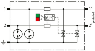
Schemata połączeń BCO ML2 BE 12
