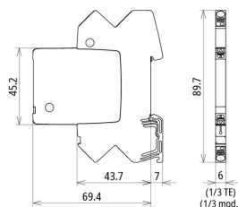
Rysunek wymiarowy BCO ML2 BE 24
