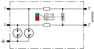
Schemat połączeń BCO ML2 BD 24
