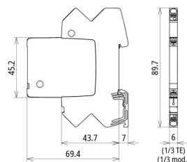
Rysunek wymiarowy BCO ML2 BE HF 5
