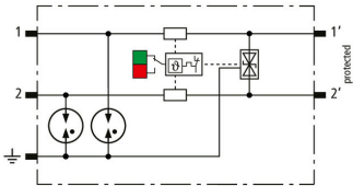
Schemat połączeń BCO ML2 BE HF 24
