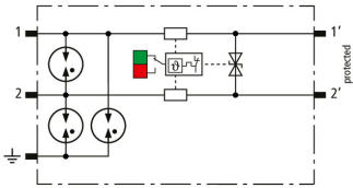
Schemat połączeń BCO ML2 BD EX 24
