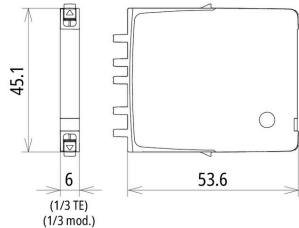
Rysunek wymiarowy BCO MOD ML2 BE 12
