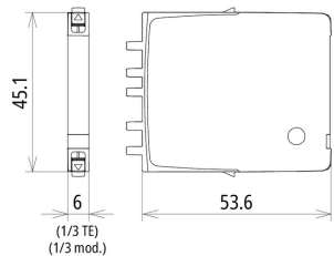
Rysunek wymiarowy BCO MOD ML2 BE 180
