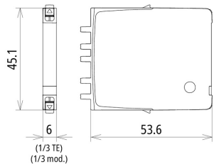
Rysunek wymiarowy BCO MOD ML2 BD 12
