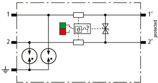
Schemat połączeń BCO MOD ML2 BD 48
