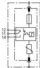
Schemat połączeń DG SE CI 440 FM
