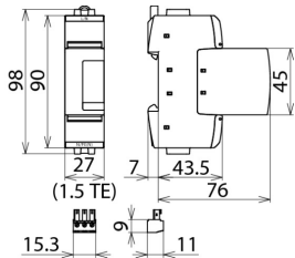
Rysunek wymiarowy DG SE CI 440 FM
