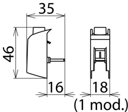
Rysunek wymiarowy STAK 25
