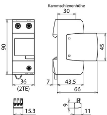
Rysunek wymiarowy DV M2 TT 2P 255 FM
