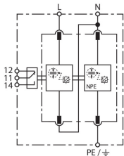
Schemat połączeń DV M2 TT 2P 255 FM
