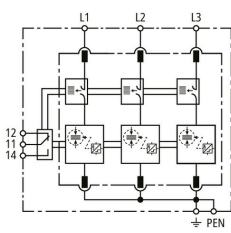
Schemat połączeń DV ACI M TNC 264 FM
