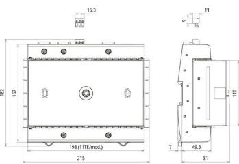
Rysunek wymiarowy DV ACI M TNC 264 FM
